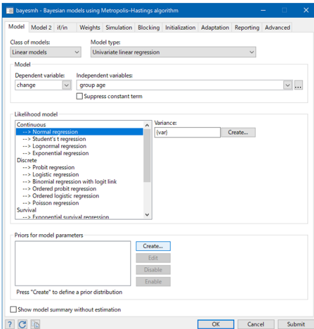
図 1 bayesmh ダイアログ - Model タブ
