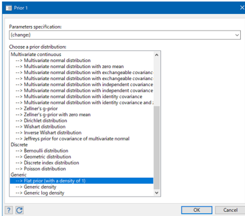
図 2 Prior 1 ダイアログ
